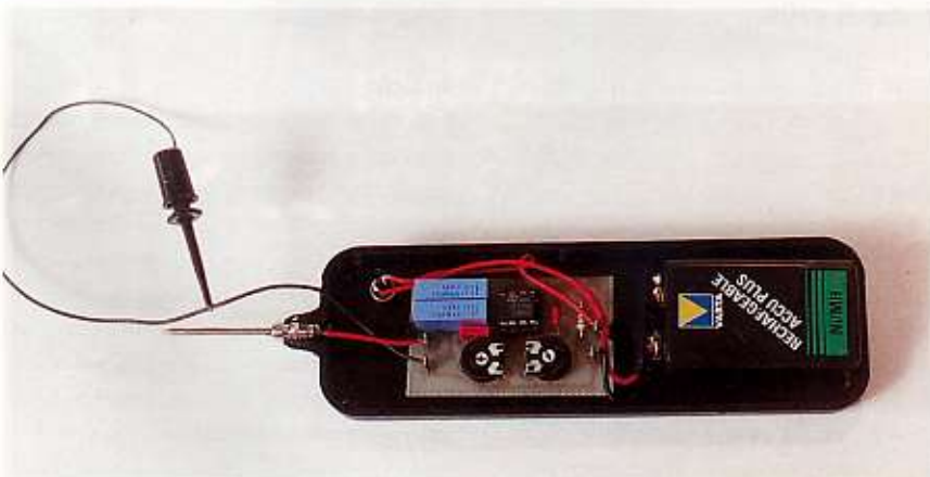
De signaalinjector in diverse stadia van afbouw.
